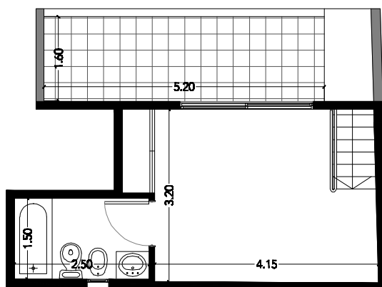
Planta Alta
