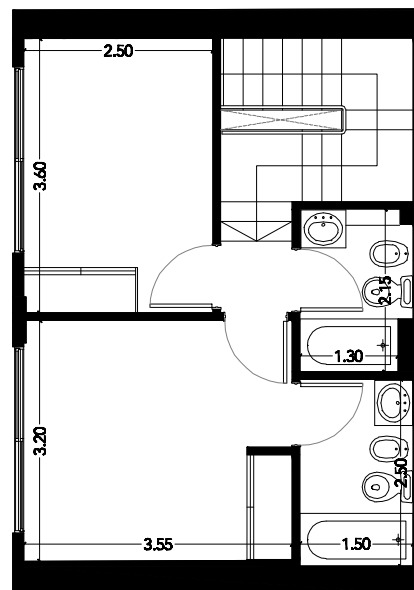
Planta Alta
