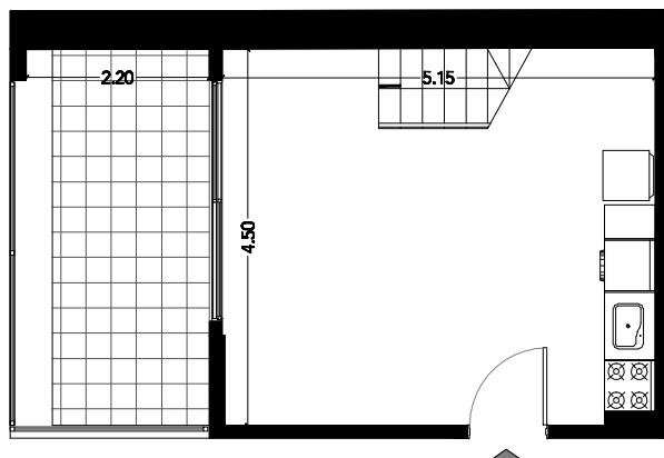
Planta Baja
