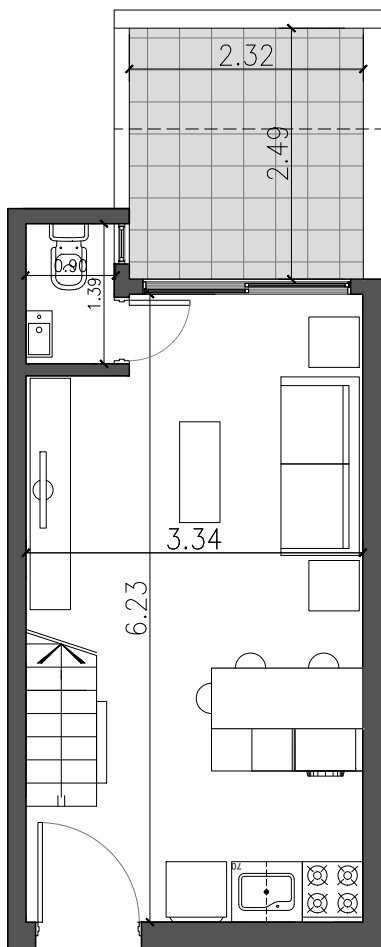
Planta baja
