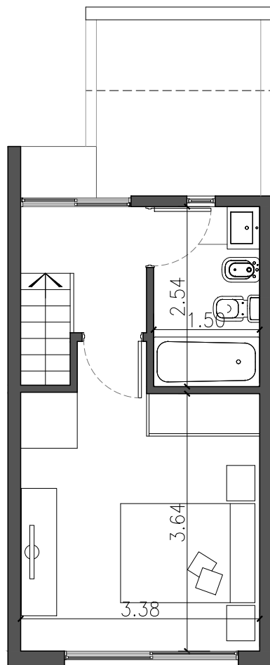
1º Piso
