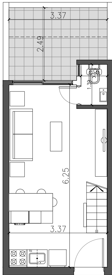
Planta baja
