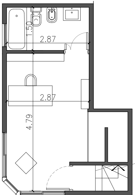
1 °Piso
