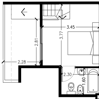
1° PISO
