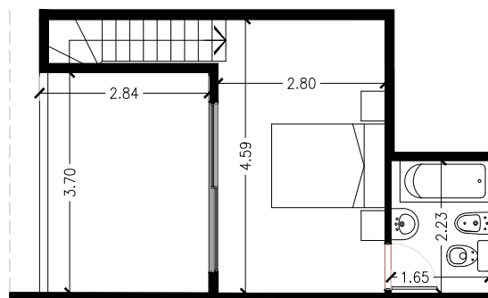
PLANTA TERCERA
