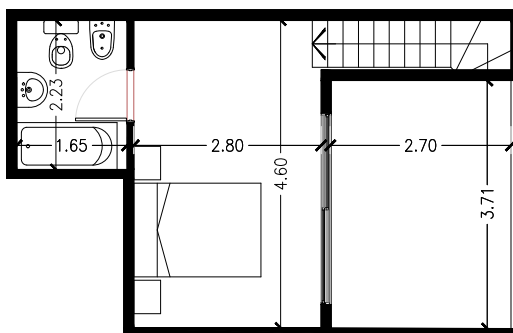
PLANTA TERCERA
