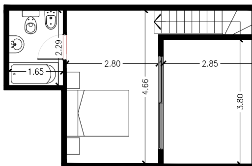
PLANTA TERCERA
