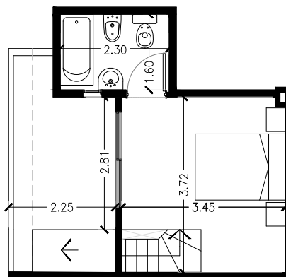
1° PISO
