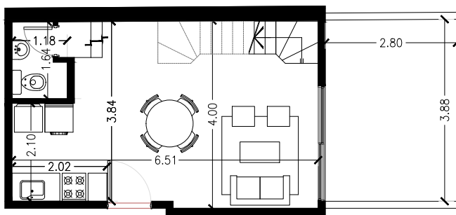
PLANTA BAJA
