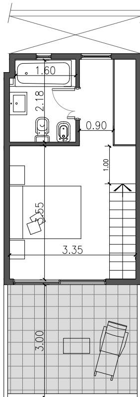
5 ºPiso
